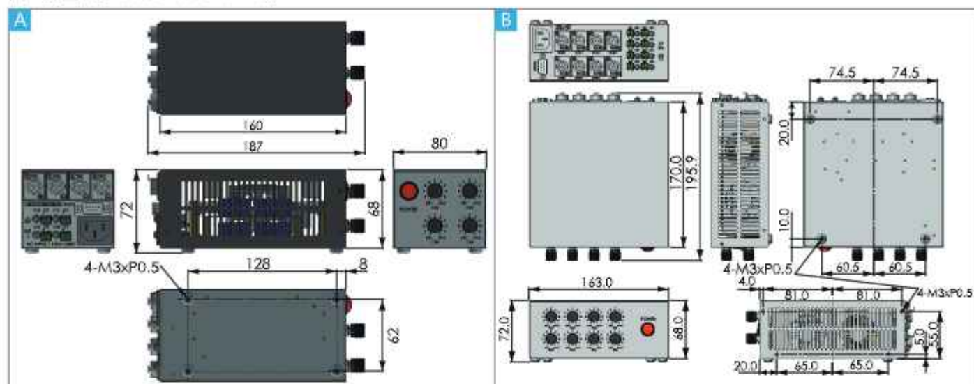
尺寸圖 (接頭樣式僅供參考)
