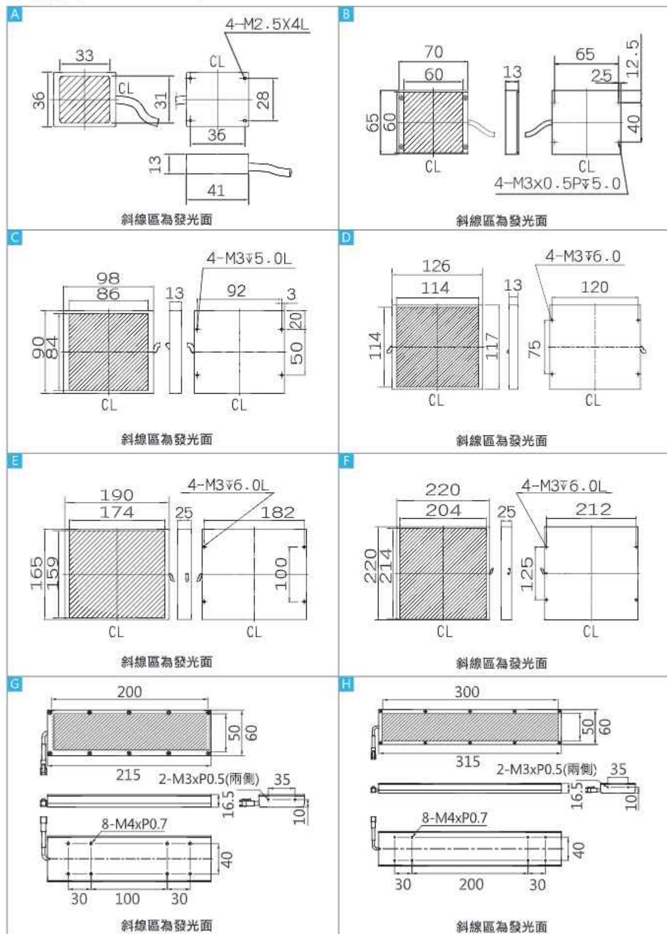
尺寸圖 (接頭樣式僅供參考)
