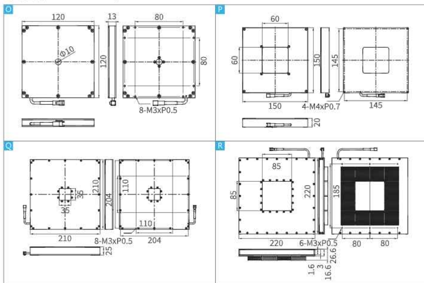
尺寸圖 (接頭樣式僅供參考)
