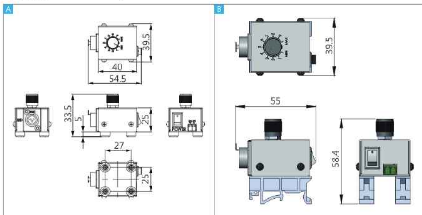
尺寸圖 (接頭樣式僅供參考)
