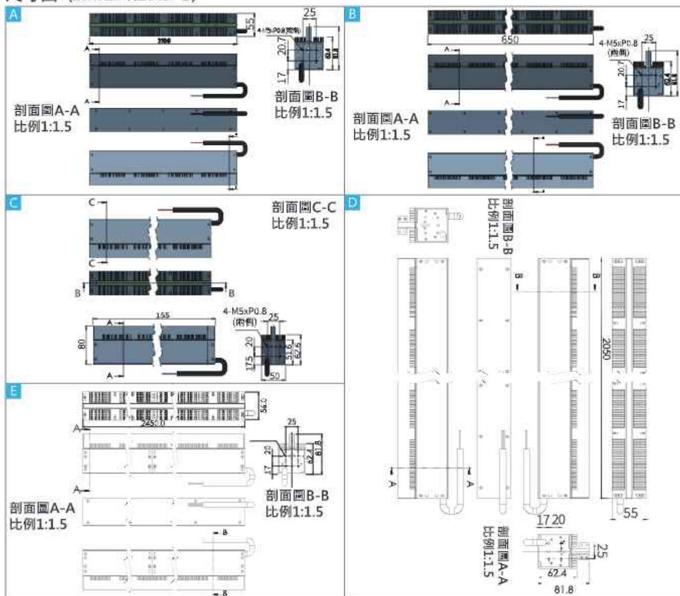
尺寸圖 (接頭樣式僅供參考)
