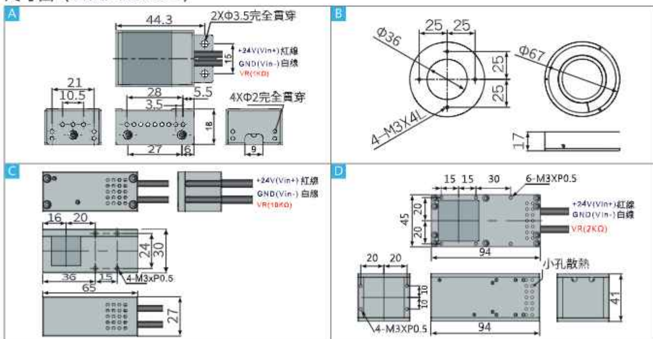
尺寸圖 (接頭樣式僅供參考)
