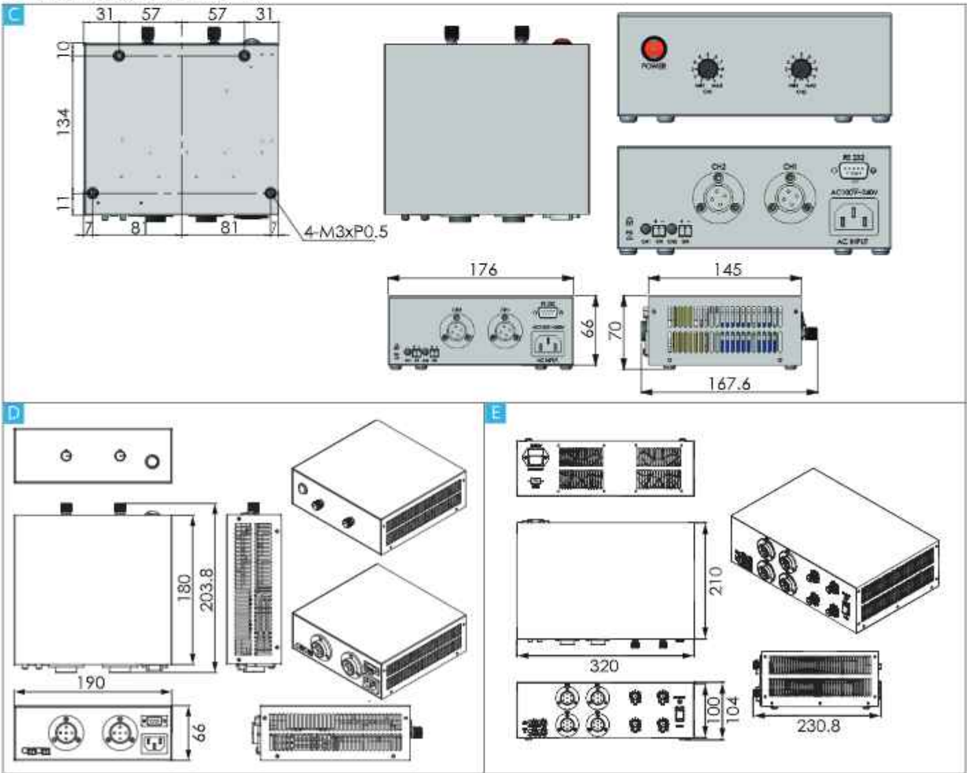
尺寸圖 (接頭樣式僅供參考)
