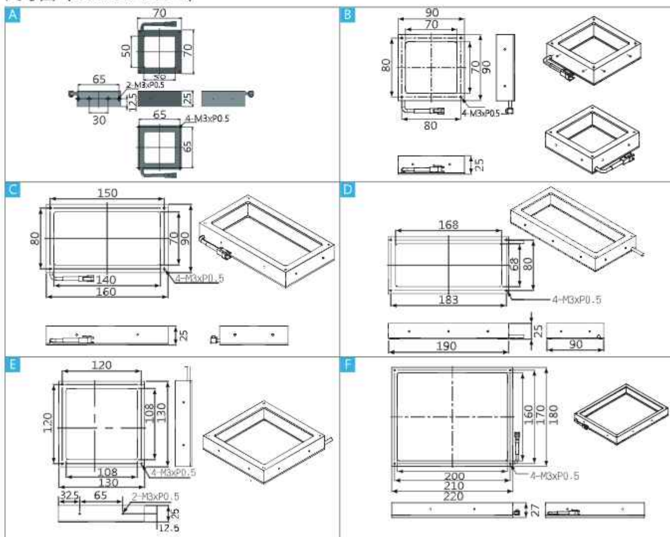
尺寸圖 (接頭樣式僅供參考)
