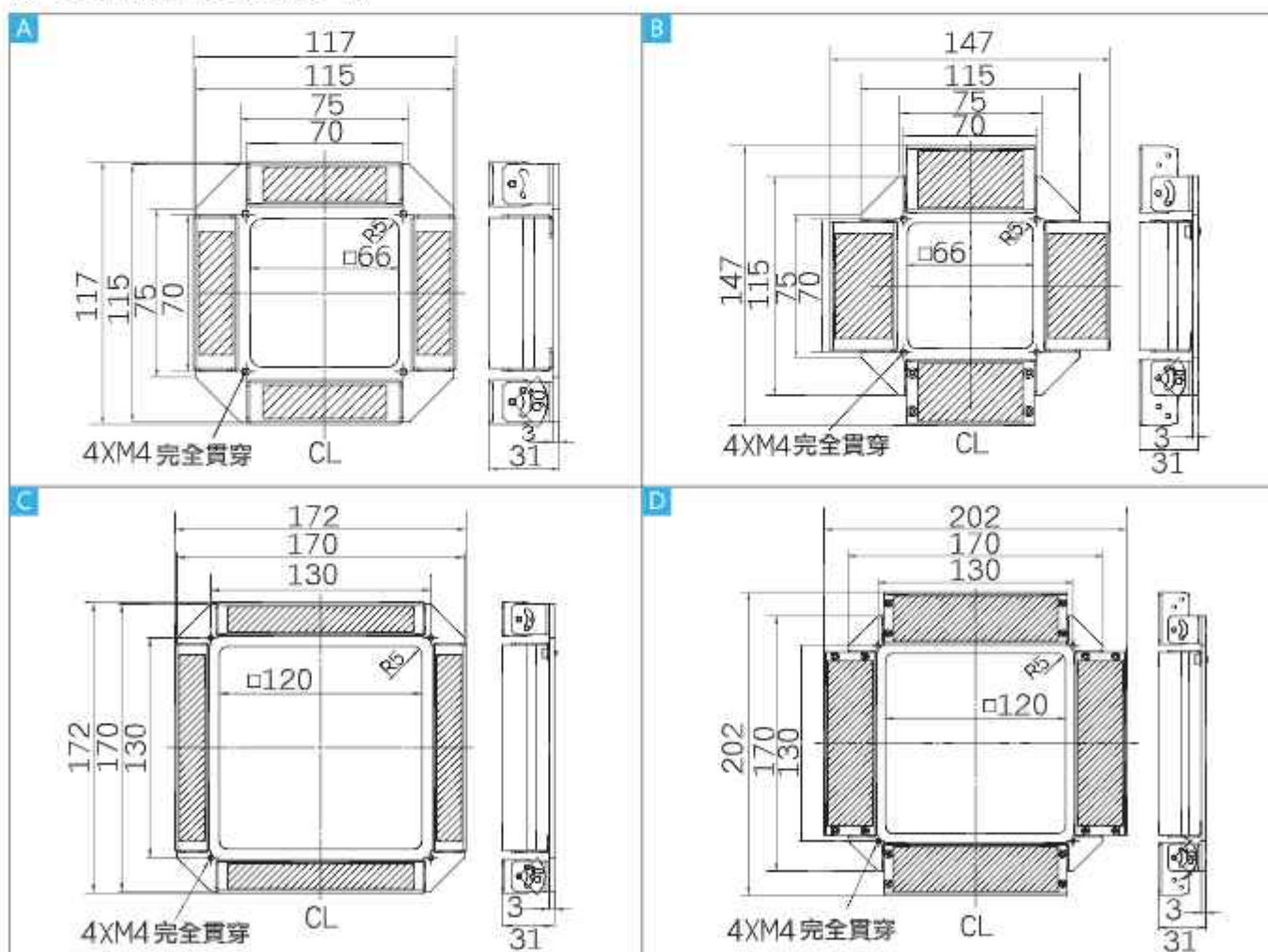
尺寸圖 (接頭樣式僅供參考)
