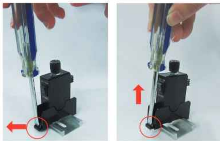
迷你軌道式定電流手動調光器拆卸方法
