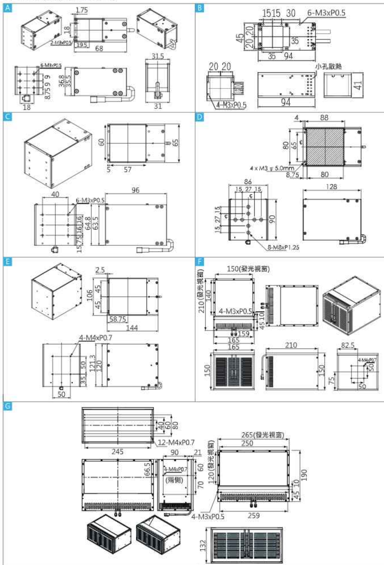
尺寸圖 (接頭樣式僅供參考)
